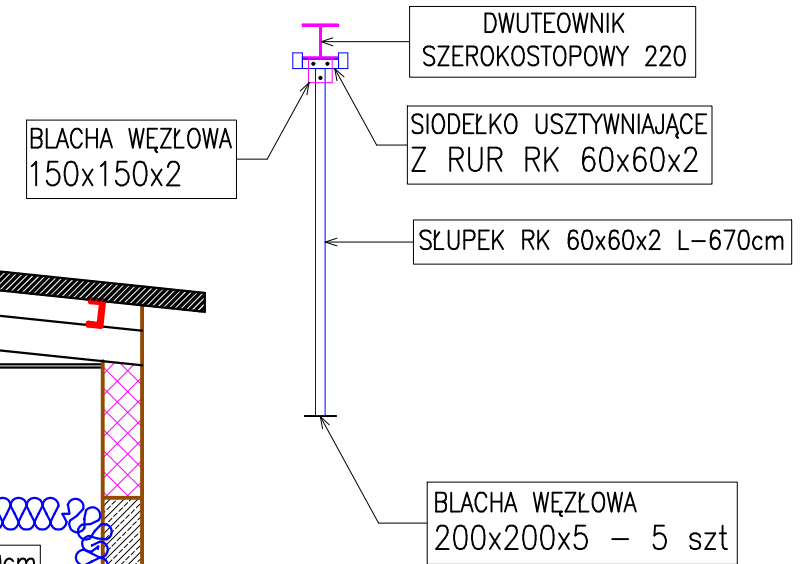
SZCZEGÓŁ "A" - SCHEMAT
